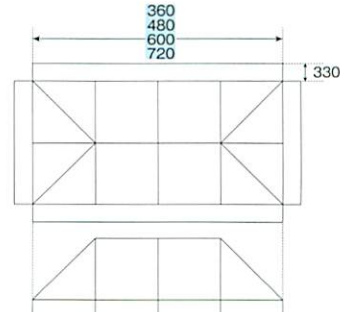
T-24(240×480) T-13(180×360) T-36(300×600) T-37(360×720)
